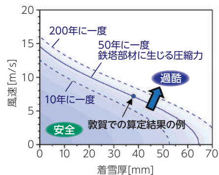
図3 送電鉄塔に対する着雪と風の過酷度評価
