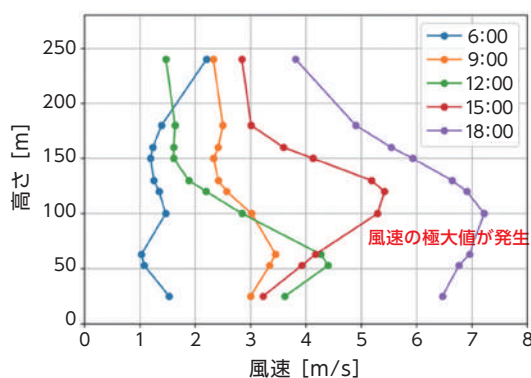
ハブ高さ付近で生じる風速極大値の発生事例(左)と洋上風況(ハブ高さ相当)の予測結果(右)
