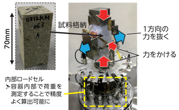
図2 減圧式真三軸圧縮試験(RTTC試験)の概要
