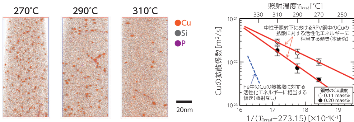
図3 照射温度によるCRC形成挙動の違い(左図)とCuの拡散係数(右図)
