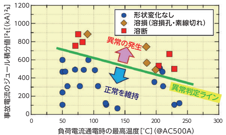
図3 負荷電流通電時の接続管温度に着目した事故電流通電時の異常判定 停電することなく圧縮形接続管の状態を把握することができ、その接続管が設置されている送電線固有の事故電流通電時に異常が発生するか否かを簡単に評価できます(図3は負荷電流が500Aの場合の診断図です)。
