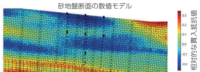
図3 傾斜砂地盤数値モデルの貫入抵抗値の補間計算例
