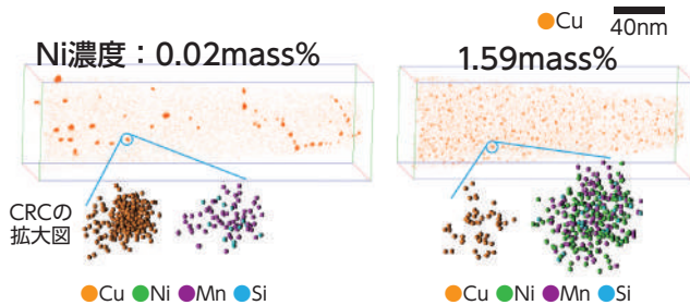
図1 鋼材のNi濃度によるCRCの形成挙動と構造の違い
