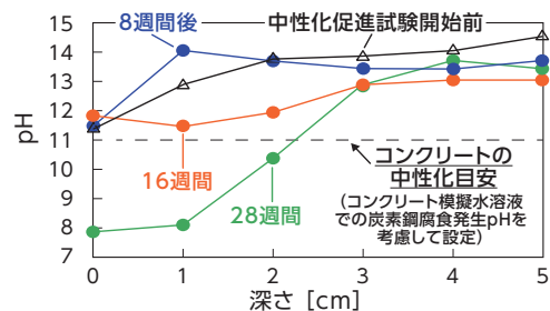
中性化促進環境下における実機材を想定したモルタル(混合材あり)供試体の深さ方向のpH測定結果(週数は中性化促進試験開始後からの期間)
