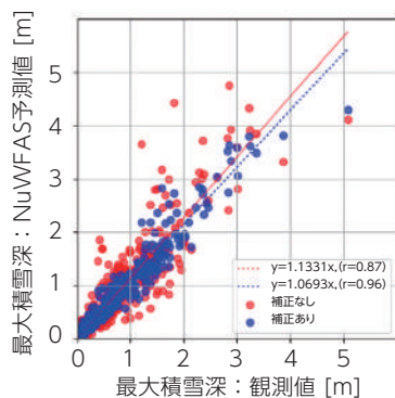
図2 最大積雪深の観測値とNuWFAS予測値の比較
