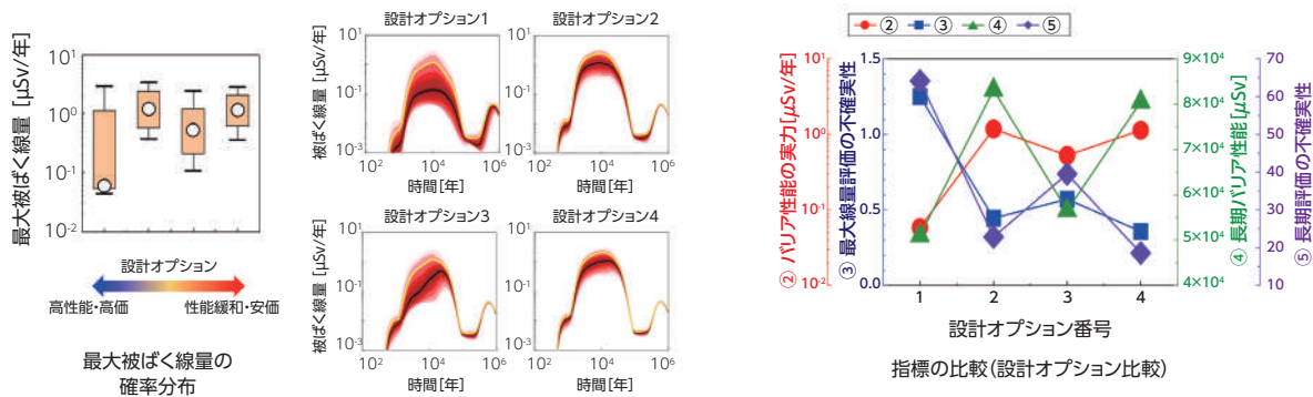
図2 中深度処分施設の設計オプションの比較評価例
