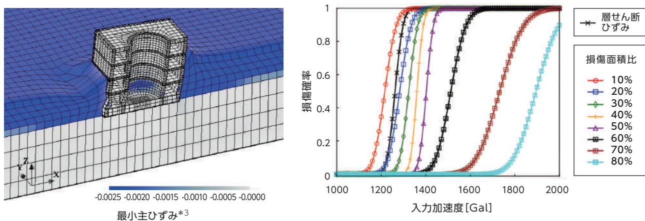
建屋 fragility の試評価 (損傷面積比に応じた fragility 曲線の変化)
