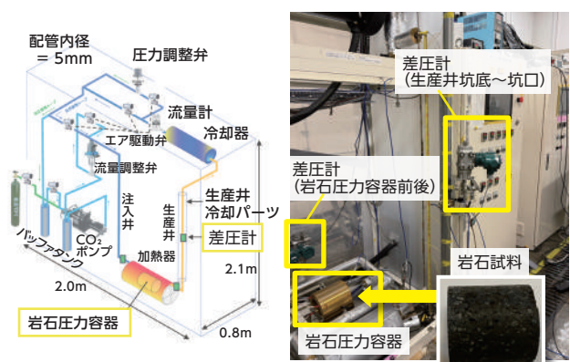
室内実験装置の外観図 (黄色い四角で囲った部分が改良箇所)
