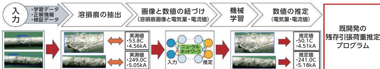
架空地線の溶損痕画像に基づく電気量および電流値の推定手法
