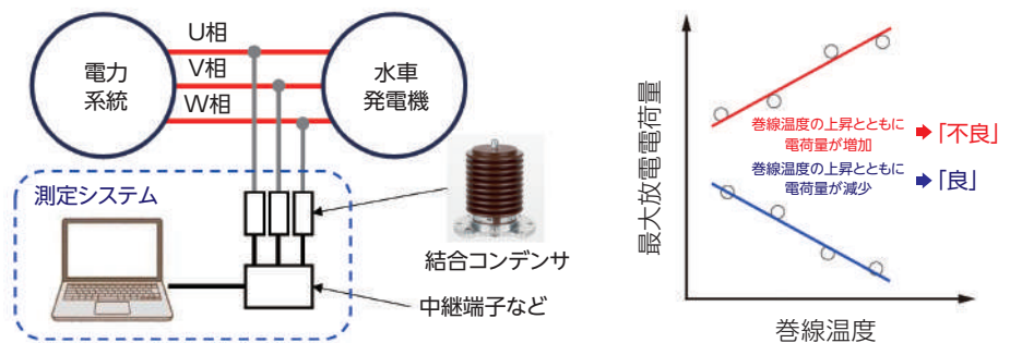
図3 運転中の部分放電測定システムの構成例(左)と簡易絶縁劣化診断手法のイメージ(右) 運転中に部分放電信号と巻線温度を計測し、最大放電電荷量との関係性を評価します。
