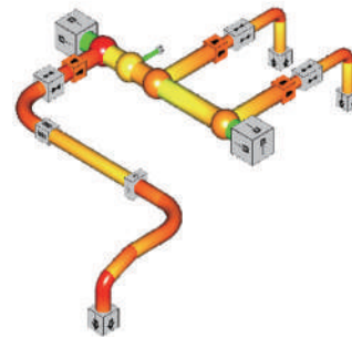
FALSETによる減肉率の評価例と提案した規格
