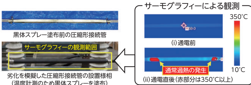
図1 事故電流通電時の圧縮形接続管の様相(電流31.5kA、通電時間0.5s)
