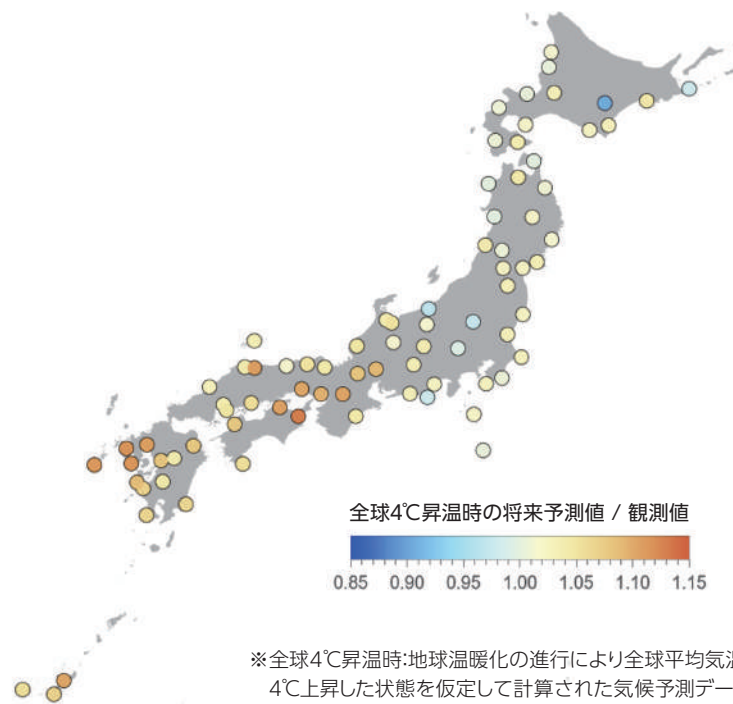
気象官署における再現期間50年の風速の将来倍率(全球4℃昇温時の将来予測値/観測値)
