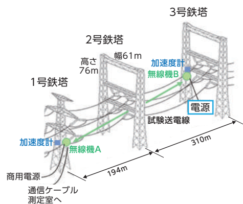
送電鉄塔周辺での利用を想定した電波伝搬試験の概要(塩原実験場 試験送電線での試験)
