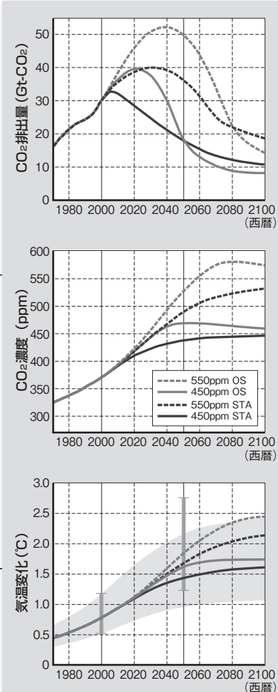
図1 450ppmおよび550ppm濃度安定化に至る経路の例
