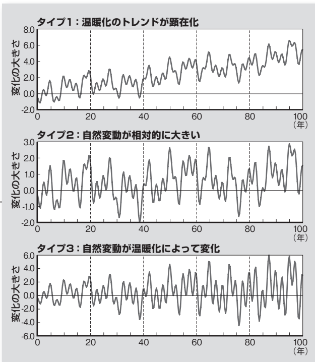
図2 人為的な温暖化トレンドと周期的な自然変動を含む概念的な気候変数の時系列
