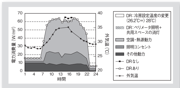
図5 モデル事務所ビルの電力負荷曲線と負荷削減量 個別電気空調、床面積5千㎡未満 (夏期平日の13～16時の間にデマンドレスポンスプログラムを発動する場合) [5]
