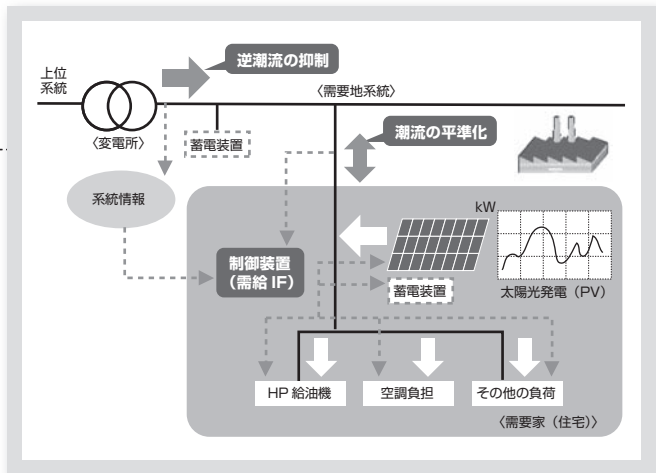
図4 需要地系統における需給一体化運用・制御
