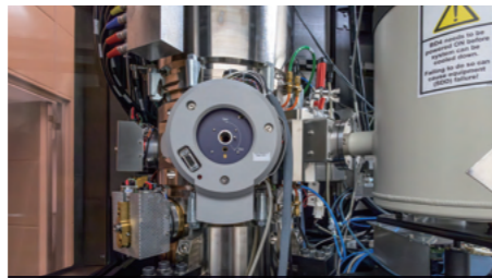
高分解能透過電子顕微鏡(収差補正TEM)
