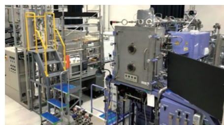
事故時燃料棒破損試験設備
