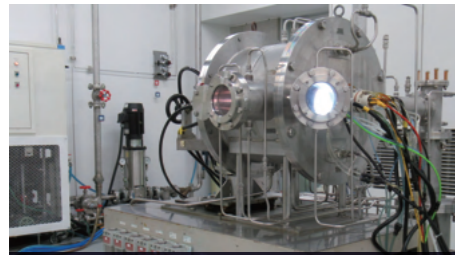
ガスタービン用遮熱コーティング(TBC)熱サイクル試験装置
